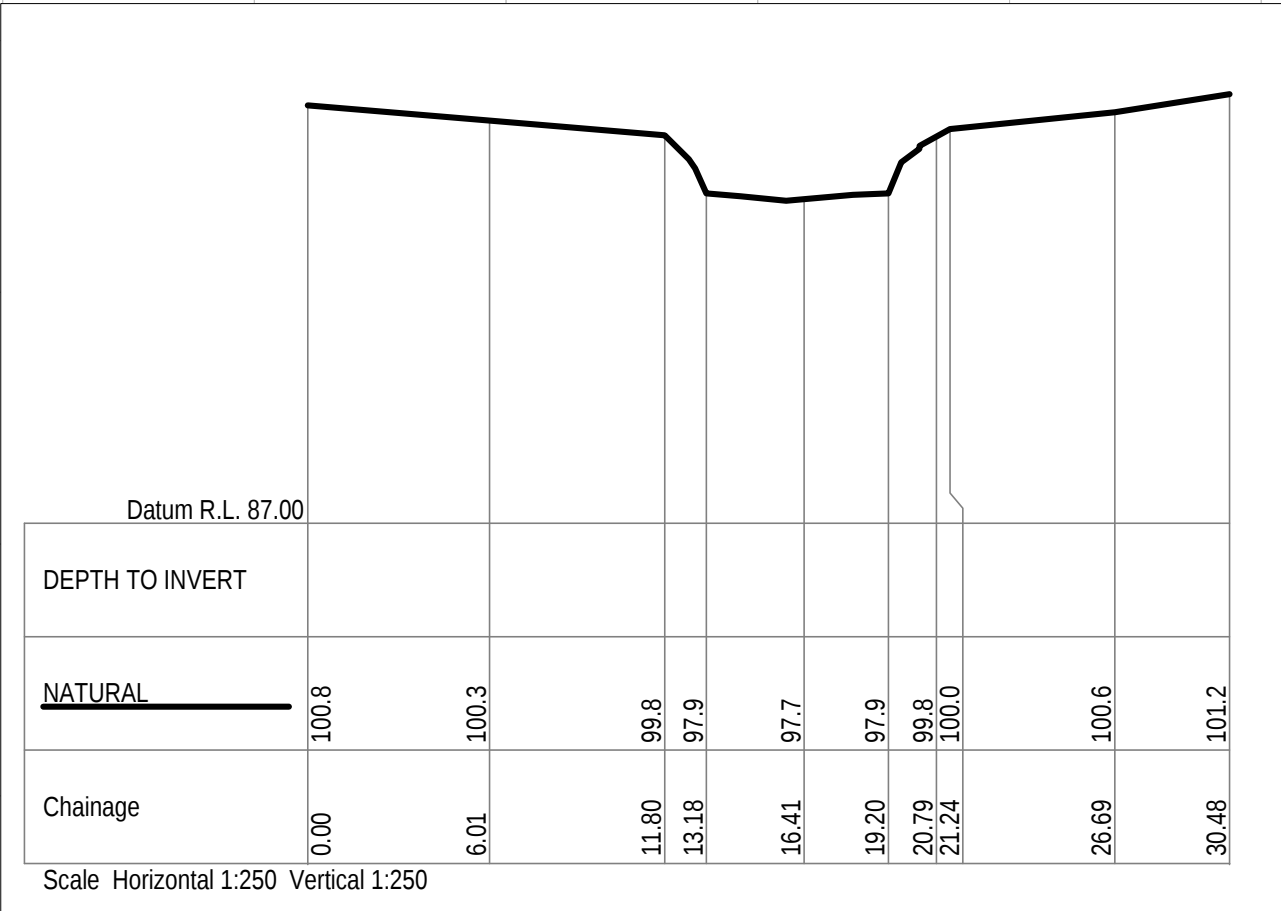
LONGITUDINAL SECTION
